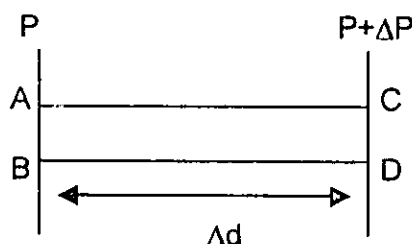
Fig. 3.2.2 Uma partícula de ar ABCD com 1\text{cm}^2 de secção entre as isóbaras P e P+\Delta P . (Meteorologia, geral e agrícola 1ª parte por F. Reis Cunha 1972)
