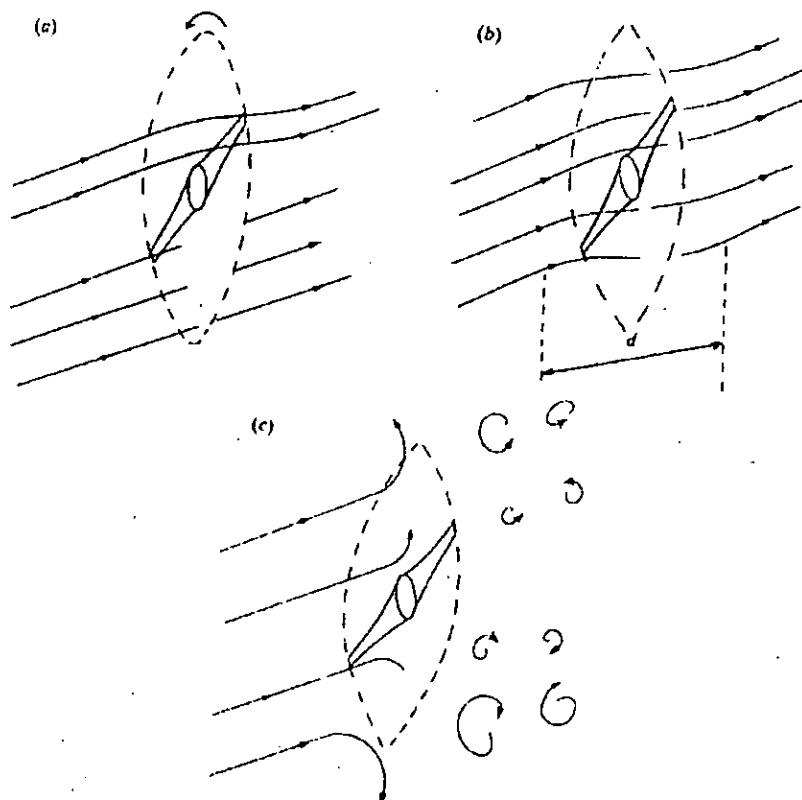
Fig.3.5.9 Mostra a frequência da turbina e a energia extraída. (a) frequência rotacional muito lenta, algum ar passa a secção menor através do disco actuador. (b) frequência rotacional óptima , todo o conjunto é afectado pelo fluxo de ar, onde d é o comprimento criado pela perturbação forte do vento pela rotação das lâminas. (c) frequência rotacional alta: A energia é dissipada na turbulência aparente e do decaimento do vórtice. (Renewable Energy Resources por John Twidell and Tony weir,1986)
