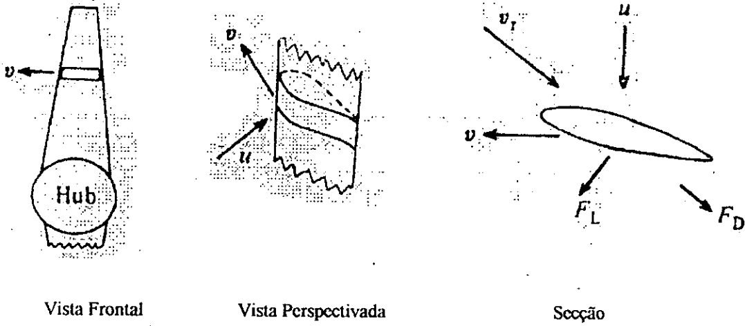
Fig. 3.5. velocidades e forças no movimento de ar nas secções das pás. Velocidades: (u) vento, (v) secção das lâminas, ( v_r ) velocidade relativa do vento na secção. Forças: ( F_D ) força de atrito em linha com ( v_r ), ( F_L ) perpendicular para ( F_D ). (Renewable Energy Resources por John Twidell and Tony weir, 1986)
