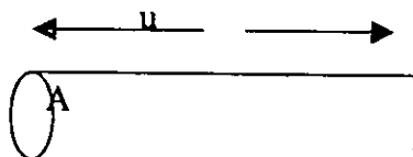
Fig.3.5.3 A massa de coluna é igual a (\rho Au) e a energia cinética é igual a 1/2(\rho Au)u^2 (Renewable Energy Resources por John Twidell and Tony weir,1986)
